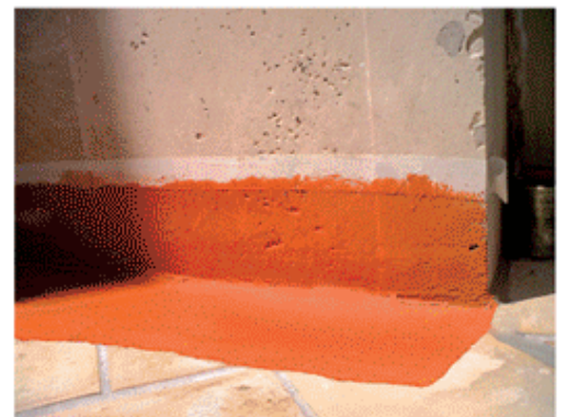
El sellado de las medias cañas se realizó con TQ CINTAFIX TEXTIL.
